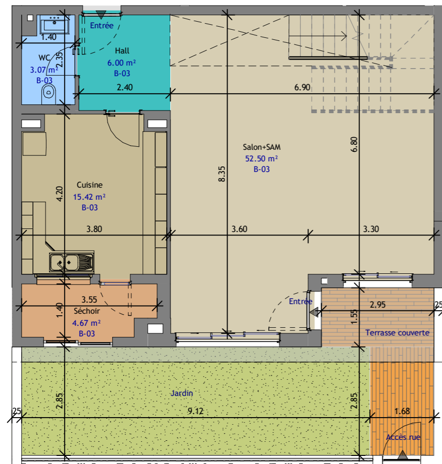
1 B-03 RDC Ech : 1 : 100
